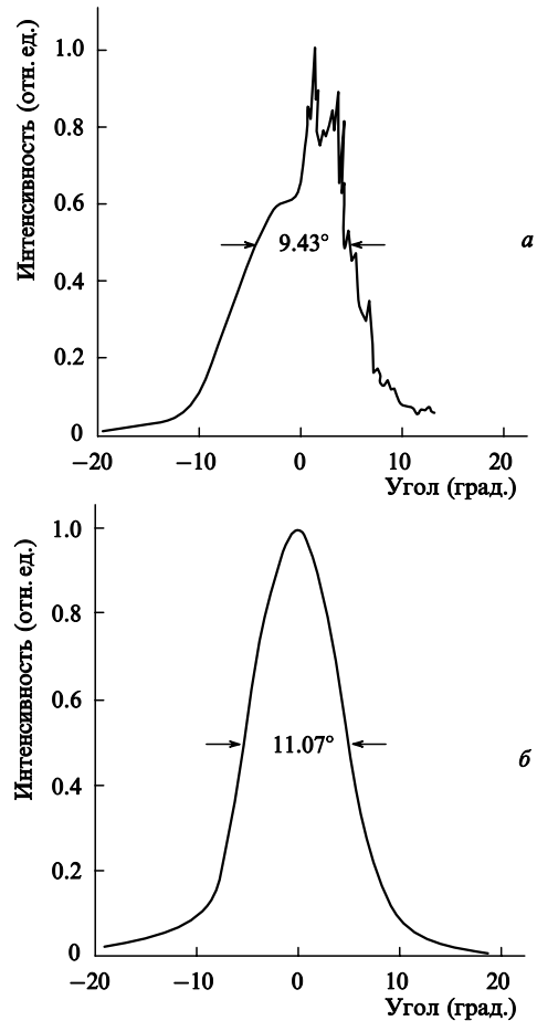
Рис.3. Распределение излучения в дальнем поле в вертикальной плоскости для ДЛ-ВИОР с шириной гребня w = 50 мкм без нанесения покрытий на оптические грани (а) и после нанесения отражающего покрытия с R_2 = 95\% на одну оптическую грань (б).
