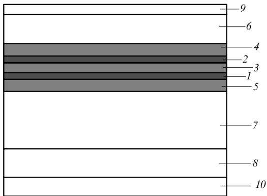
Рис.1. Схема простейшей конструкции гетероструктуры для ДЛ-ВИОР: 1, 2 – активные слои из InGaAs; 3, 4, 5 – барьерные слои из GaAs; 6 – ограничительный слой ( p -типа); 7 – слой вытекания; 8 – отражательный слой ( n -типа) для вытекающего излучения; 9 – контактный слой p + -типа; 10 – подложка n -типа из GaAs.
