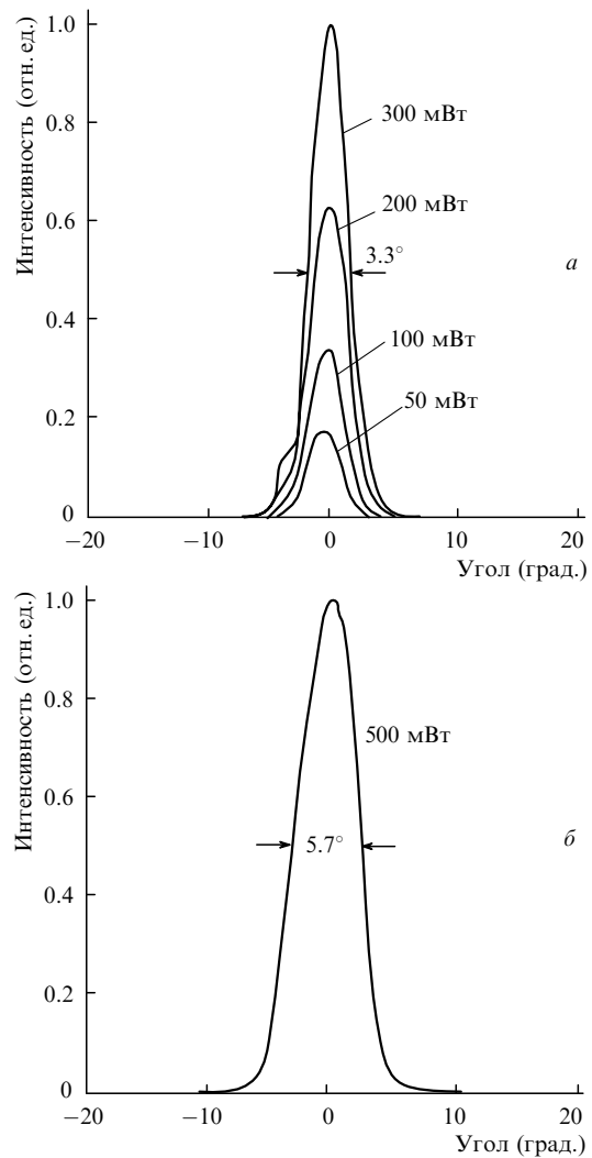
Рис.7. Распределение излучения в дальнем поле в горизонтальной плоскости для ДЛ-ВИОР с w = 10 мкм, L_{cav} = 1600 мкм, R_1 = 95\% , R_2 = 7\% при мощности излучения от 50 до 300 мВт (а) и 500 мВт (б).
